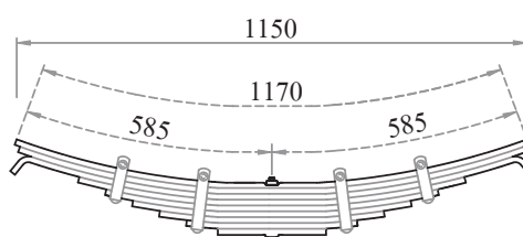
ແຜນບຂ່ວງກລາງ 3 ເຟລາ ປລາຊອ 2 ດ້ານ
