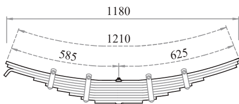
ແຜນບໜ້າ/ຫຼັງ ປລາຊອດ້ານເດີຂວ
