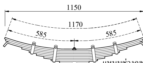
แหนบช่วงกลาง 3 เพล ปลายงอ 2 ด้าน
