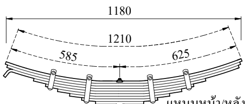
แหนบหน้า/หลัง ปลายงอด้านเดียว
