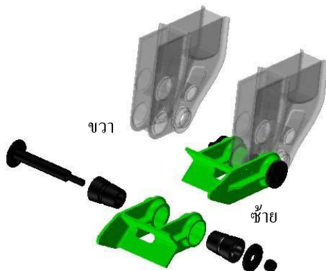
66-2140 สลัก/น็อต/แหวน โด่งตรงกลาง (ชิ้นส่วนอ้างอิงชุดสลักโด่งตรงกลาง)
